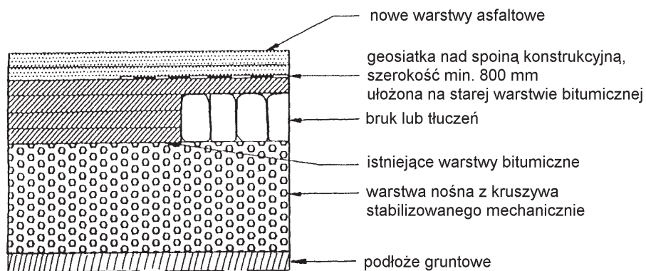
Rys. 5. Wzmocnienie nawierzchni asfaltowej w strefie poszerzenia nawierzchni
