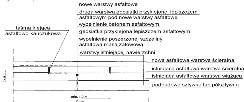
Rys. 2. Naprawa płytka pojedynczego pęknięcia odbitego, gdy krawędzie pęknięcia są dobrze podparte - w istniejącej warstwie ścieralnej, z ułożeniem nowej warstwy asfaltowej
